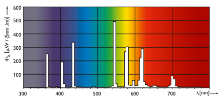
HPL 4 /634
